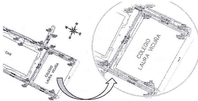
Redes de alcantarillado FASE II "CAM". Fuente: Propia
