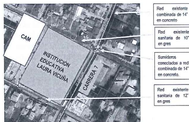
Redes existentes en calle 11 y 12 desde carrera 7A a carrera séptima. Fuente: Propia.
