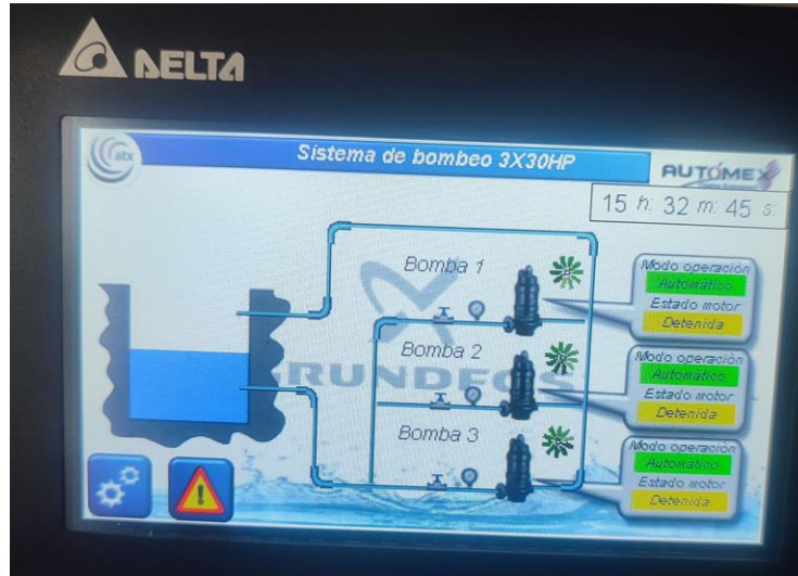
Ilustración 40. Vista Pantalla Digital de Programación bombeo RAS 1 (Reactor 1 y 2)
